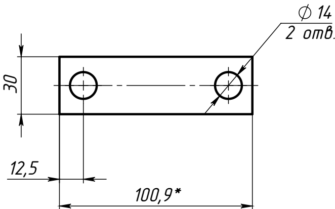
Поз.3 (Полухомут) развертка
