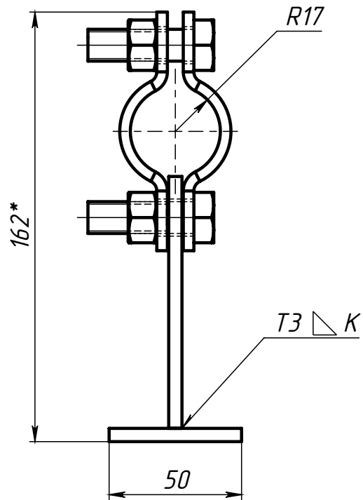
Поз.3 (Полухомут)
